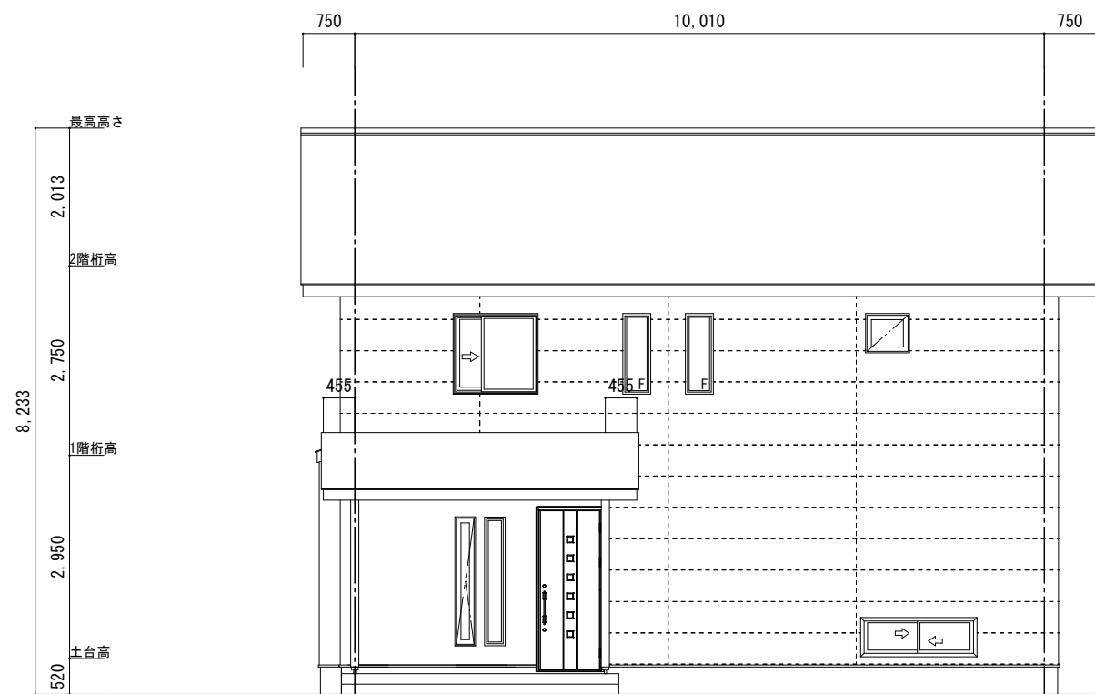
北側立面图
