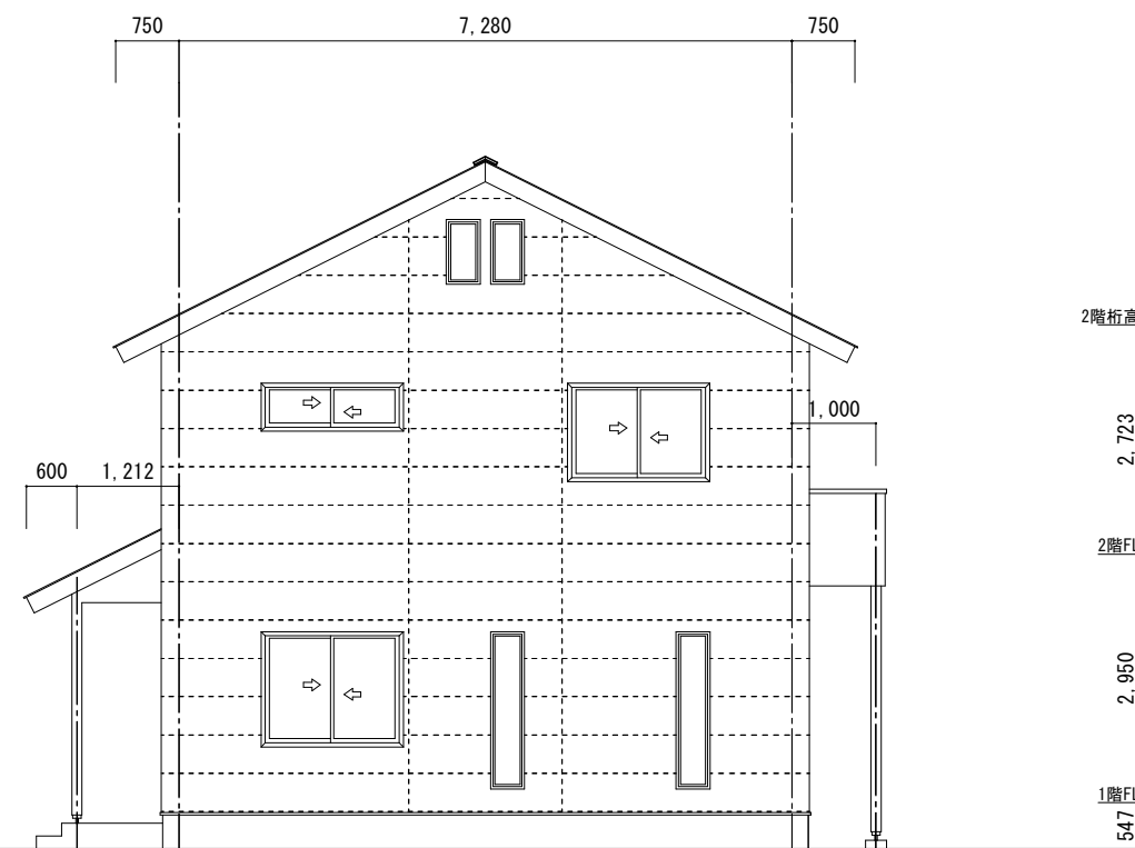
西側立面图
