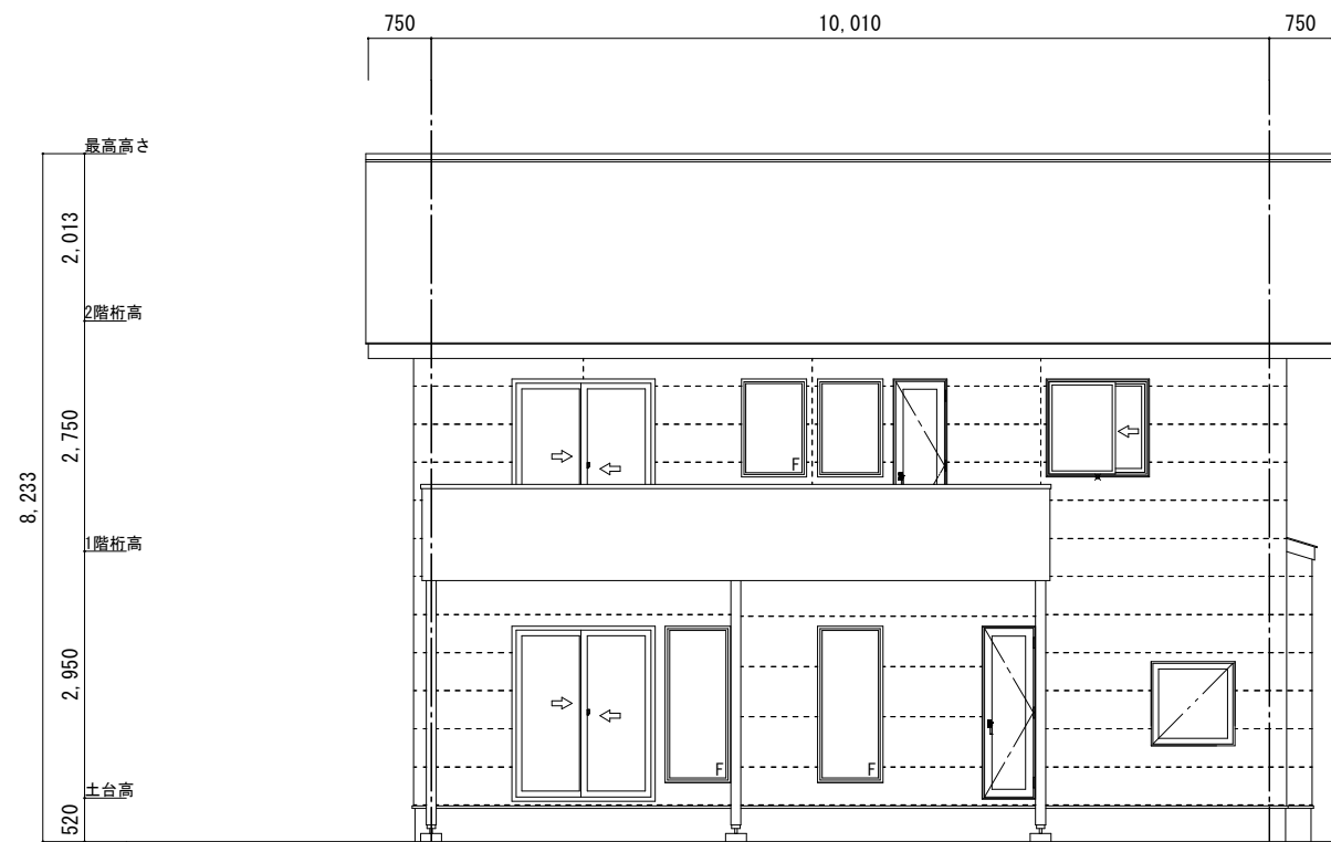
南側立面图
