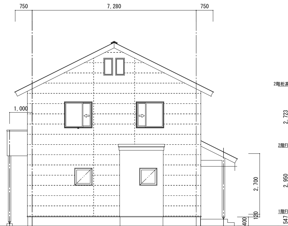
東側立面图
