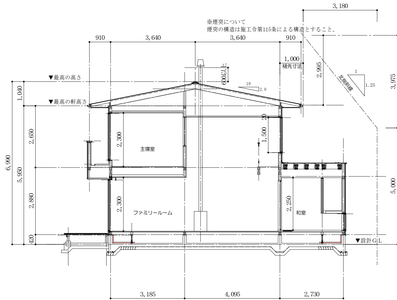
南北方向断面図
