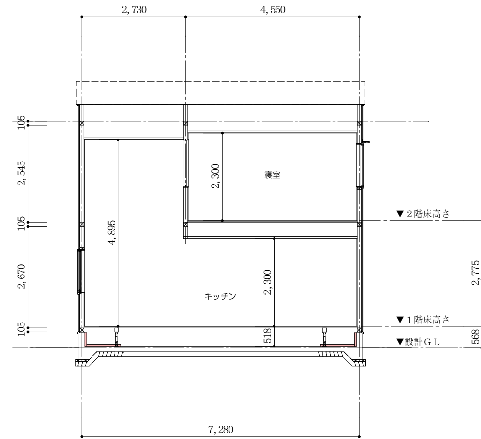
東西方向断面図
