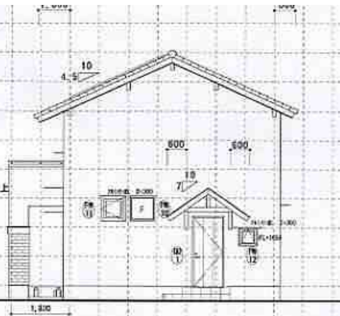
东侧立面图
