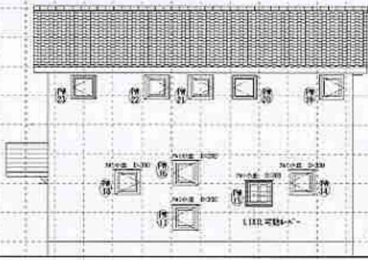
北侧立面图
