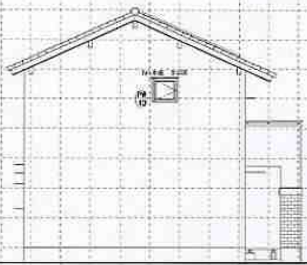
西侧立面图
