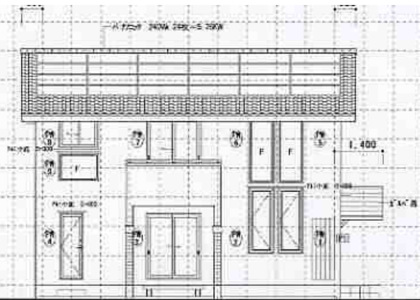
南侧立面图
